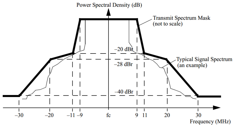
图 5.2.1-2 802.11 发射机频谱辐射模（20MHz 带宽）
