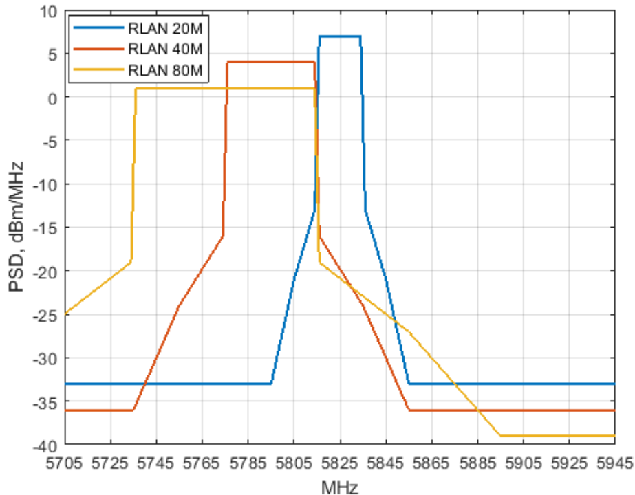
图 5.2.1-3 RLAN 不同带宽的 PSD 示意图
