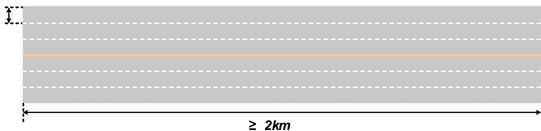
图 5.1.1-1 高速场景拓扑
