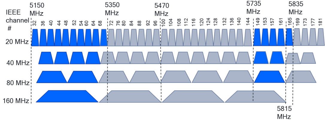
图 5.2.1-1 RLAN 信道划分示意图
