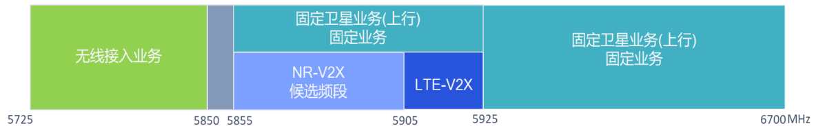
图 5-1 5.9GHz 频谱分配情况
