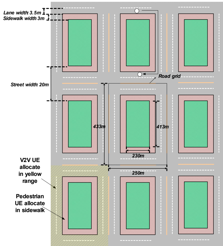
图 5.1.1-2 城区场景拓扑
