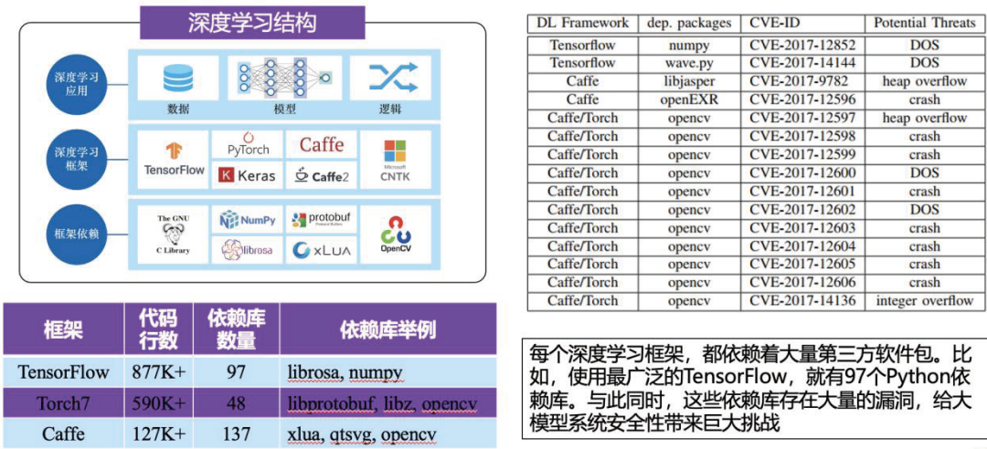
图 3-6 生成式 AI 学习框架面临的安全问题示意图
