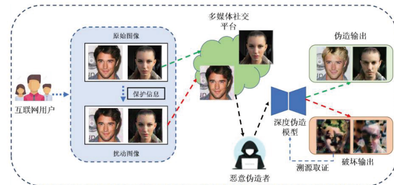
图 3-16 深度伪造主动防御技术流程图
