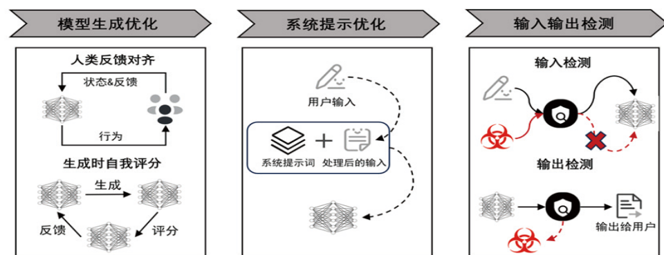
图 3-10 模型越狱防御技术的方法示意图
