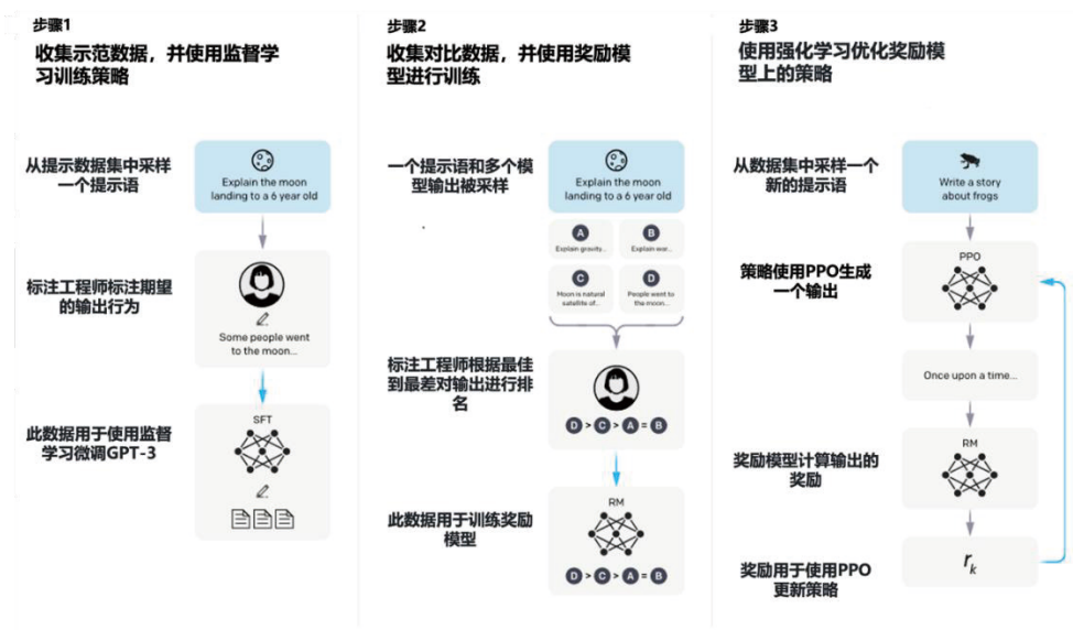
图 3-13 基于人类反馈的强化学习方法示意图
