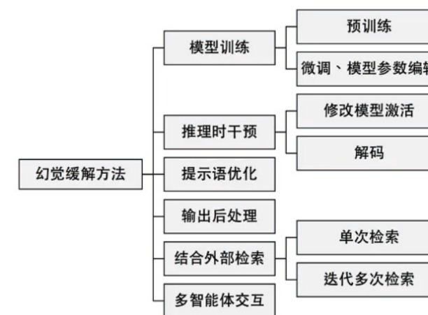
图 3-17 模型幻觉防御技术
