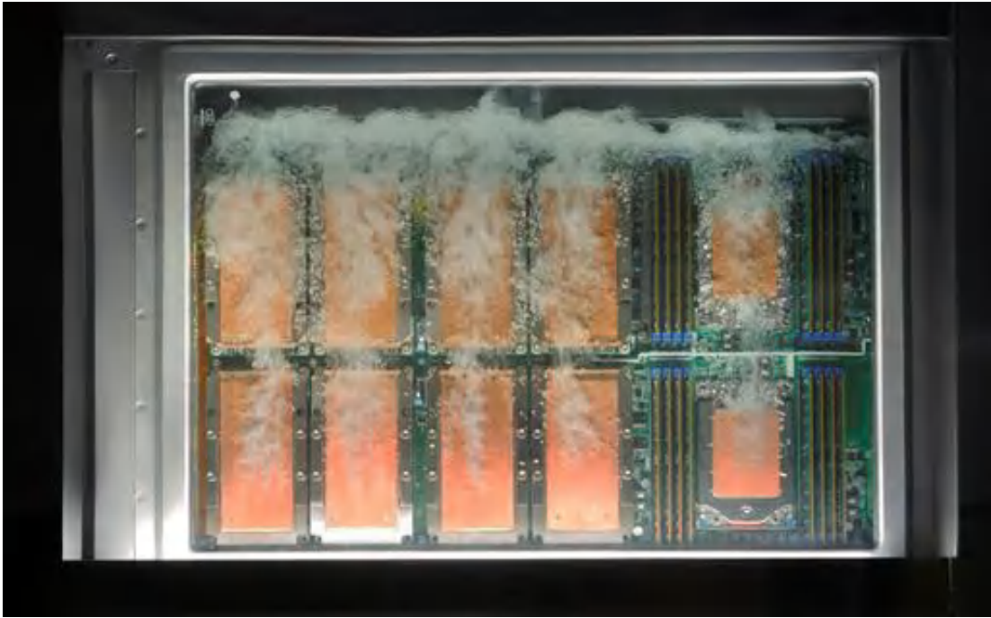
曙光相变液冷技术
